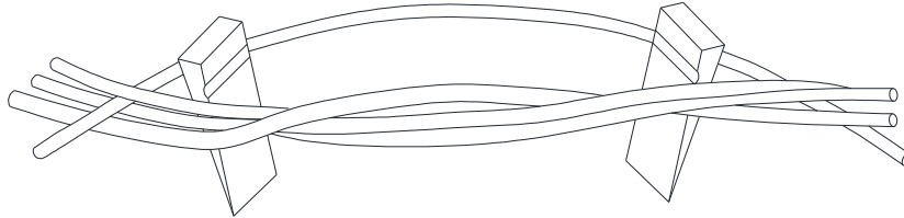
Figura 51 – Aplicação de cunha separadora
