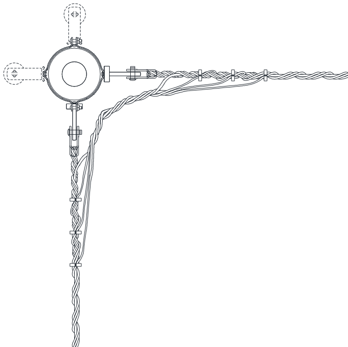
Figura 27 – Estrutura 90° - SI3 – SI3
